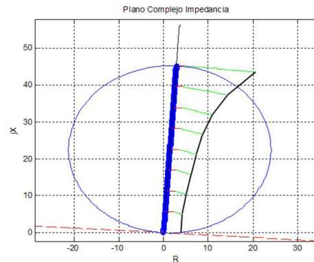
Figura 10: Error en la medición debido a la resistencia de falla ante una característica tipo MHO.
